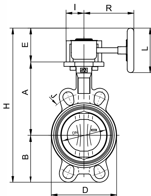
Основные параметры дискового поворотного затвора «Гранвэл» межфланцевого с редуктором
