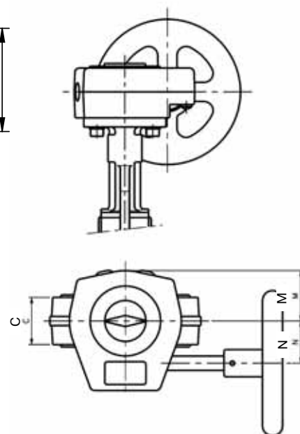
Основные параметры дискового поворотного затвора «Гранвэл» межфланцевого с редуктором
