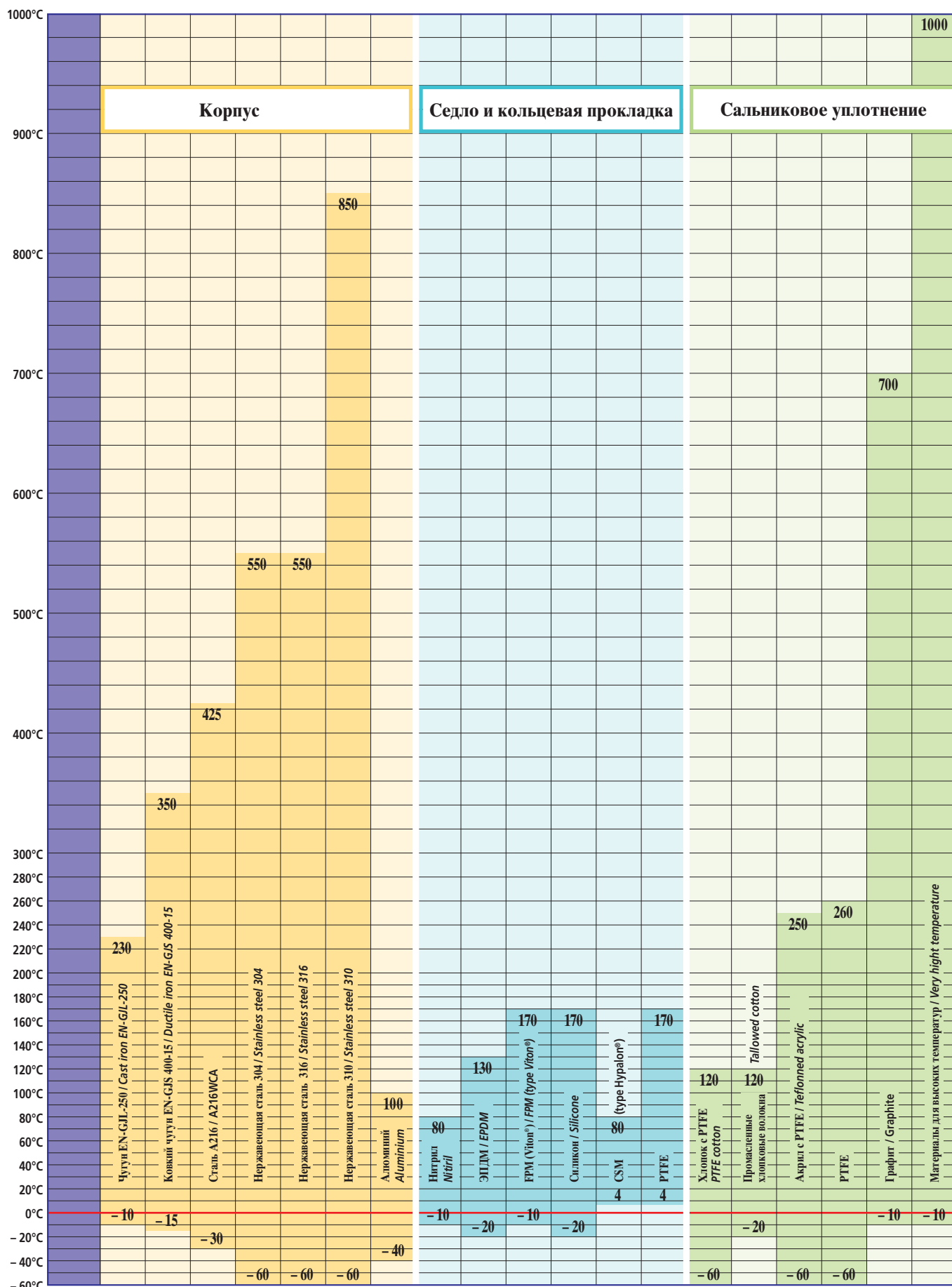
Основные материалы конструкции при производстве шиберов. Данные только для информации. Другие исполнения под заказ.
