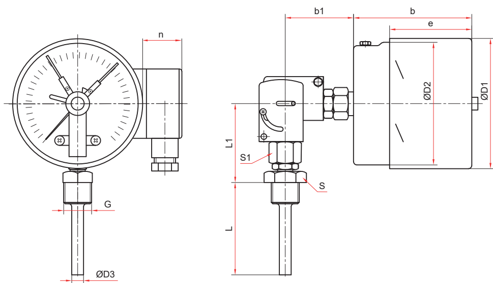
Универсальное присоединение
